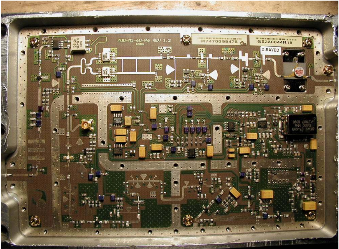
Downconvert Module
