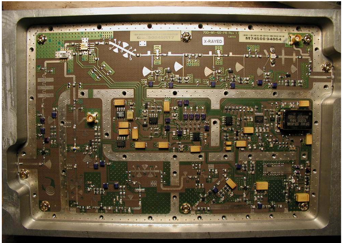
Upconvert Module
